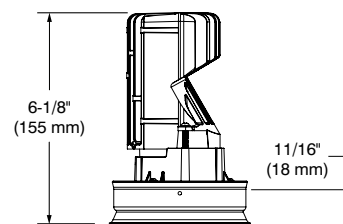
FLANGELESS TRIM
